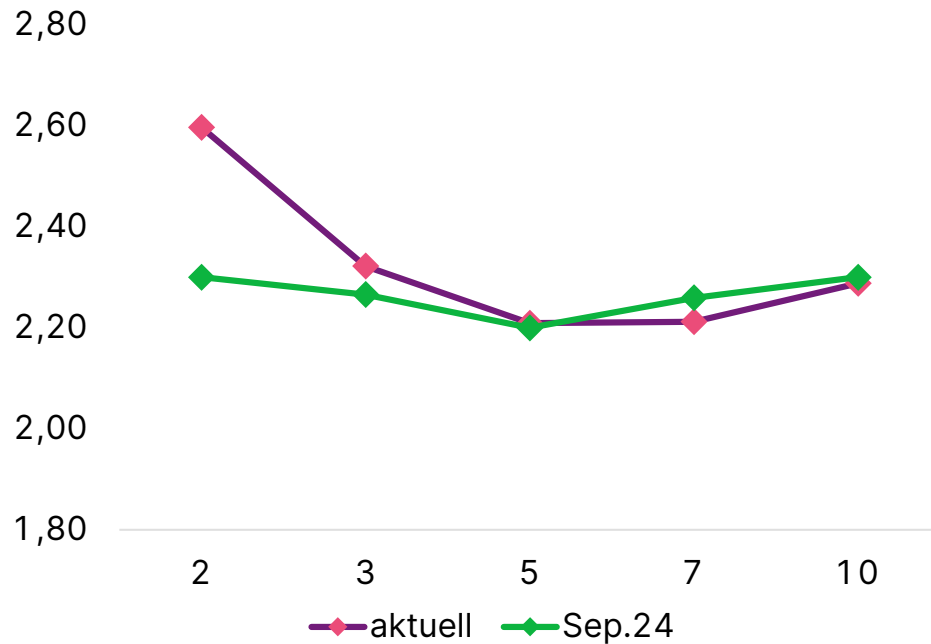
Deutsche Renditestrukturkurve (%)
