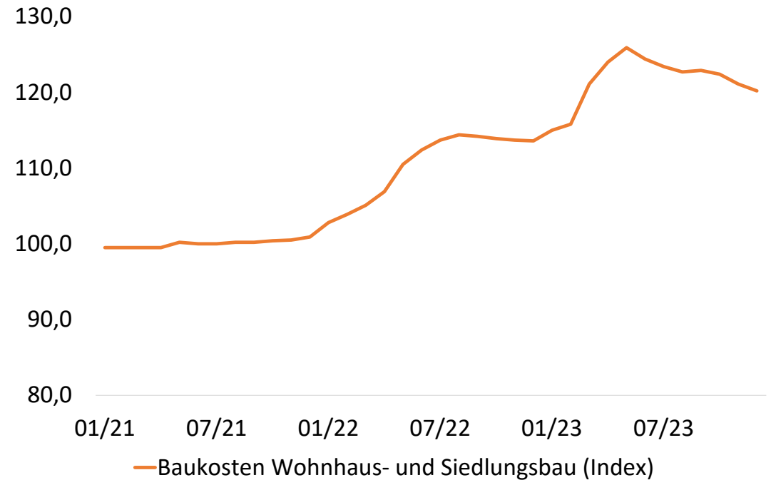
Baukosten Wohnhaus- und Siedlungsbau (Index)
